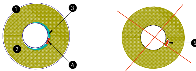
[ABB. 27] Dämmung über Begleitheizung dimensionieren.
