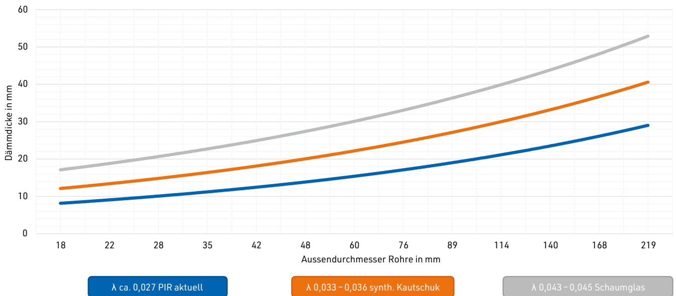
[ABB. 20] Empfohlene Dämmdicken nach Temperatur und λ-Wert.
