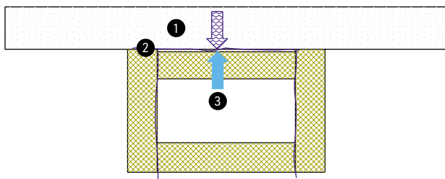
[ABB. 16] Kondensatansammlung zwischen feuchter Betondecke und Dämmung wegen Taupunktunterschreitung infolge von fehlendem Luftaustausch zwischen Decke und gedämmter Lüftungsleitung. 1 Feuchter Beton 2 Kondenswasserbildung 3 Kalte Luft
