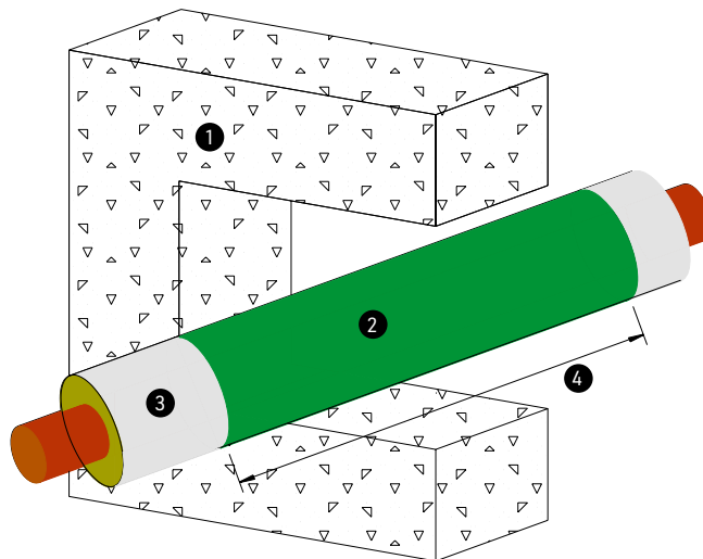
[ABB. 13] Möglicher Dämmbau im Bereich des Brandabschnitts.
