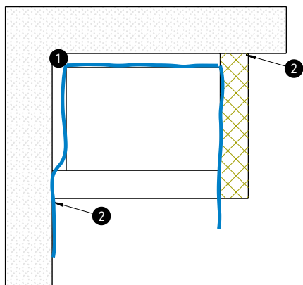
[ABB. 15] Beispiel einer Kondensatansammlung infolge Taupunktunterschreitung nicht gedämmter Lüftungsleitungen. 1 Mögliche Tauwasserbildung und Ansammlung von Wasser 2 Mögliches Eindringen von feuchter Luft
