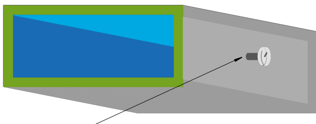
Dämmung von Fühler- und Thermometerstutzen im Tauwasserbereich mit synth. Kautschuk von mind. 13 mm Dicke.
