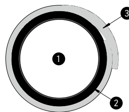
[ABB. 28] Dämmsystem gegen Tauwasserbildung inkl. Schalldämmung. 1 Rohr 2 Dämmung aus Kautschuk (gegen Schwitzwasser) 3 Schwerfolie (Schalldämmung)
