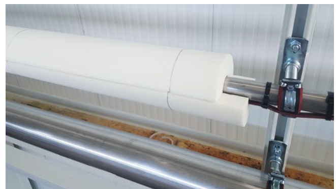
[ABB. 8] Versetzt angeordnete Dämmung mit Kunststoffhalbschalen aus Polyisocyanurat (PIR).
