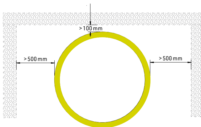
[ABB. 6] Mindestabstand zwischen gedämmtem Behälter und Bauteil oder anderen Installationen.
