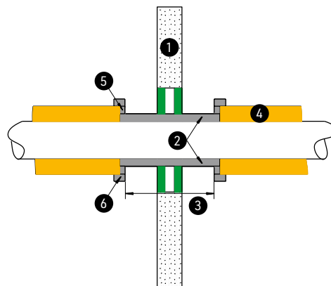
[ABB. 30] Mögliche Ausführung von Brandabschnittsdurchführungen. 1 Brandabschnittsbildendes Bauteil 2 Geprüfte Streckendämmung durch Brandabschnitt 3 Länge der geprüften Streckendämmung 4 Kälteführendes Dämmsystem 5 Aufdoppelung mit Material der geprüften Streckendämmung 6 Deckstreifen aus Material der geprüften Streckendämmung mit L > 100 mm
