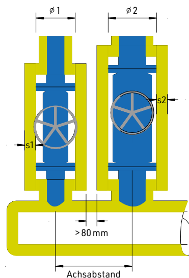
[ABB. 3] Minimalabstände zwischen gedämmten und nicht gedämmten Rohrleitungen.
