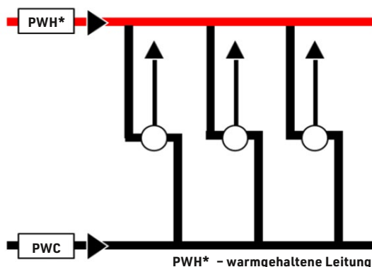
[ABB. 6] Mögliche Darstellung neuralgische Stelle Duschen.
