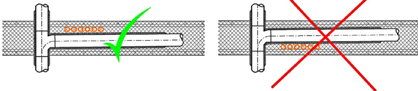
[FIG. 2] Incroci con tubo di scarico. (Immagine: Alco Haustechnik AG)
