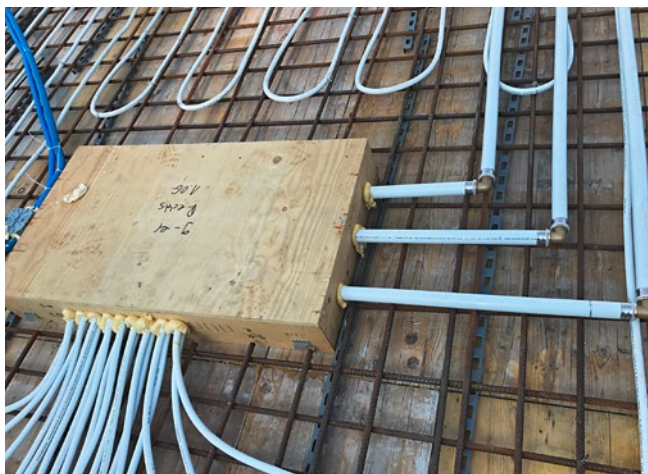
[FIG. 3] Esempio di una scatola da incasso per distributori TABS.
