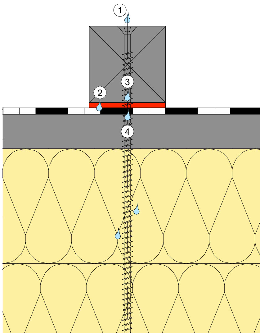
[FIG. 1] Possibili aree di infiltrazione dell'umidità nei punti di penetrazione dei fissaggi nei sottotetti. 1 Infiltrazione dalla testa della vite 2 Infiltrazione attraverso la guarnizione punto chiodo 3 Infiltrazione al di sopra della guarnizione punto chiodo 4 Infiltrazione al di sotto della guarnizione punto chiodo
