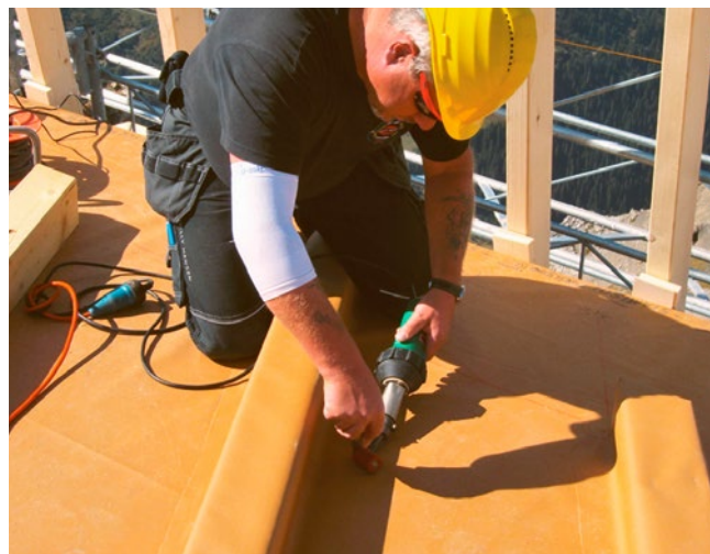
[FIG. 3] Sigillatura completa del controlistello con membrane saldate.
