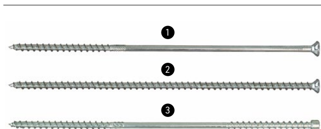
[FIG. 8] Tipi di filettatura: 1 Vite parzialmente filettata 2 Vite interamente filettata 3 Vite con doppia filettatura
