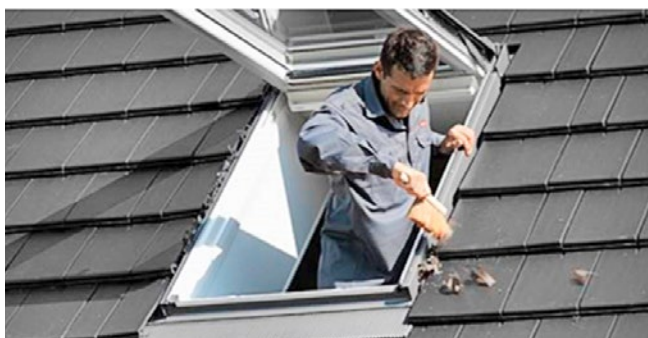
[FIG. 2] Elevato rischio di infiltrazioni d'acqua nei raccordi a causa dell'accumulo di sporcizia.
