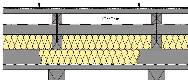
[FIG. 6] Combinazione di posa non omogenea (sopra) e omogenea (sotto).
