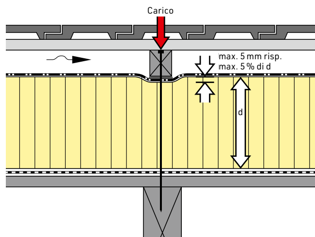
[FIG. 7] Deformazione massima pari al 5% dello spessore totale, non superiore ai 5 mm.
